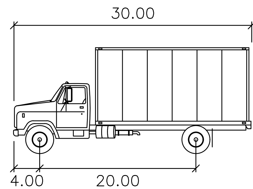
SU-30
